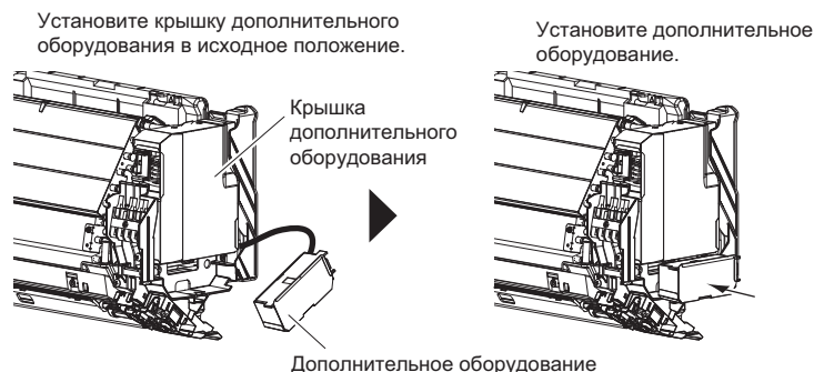
Рис. 3. Установка дополнительного оборудования
