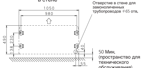
Расположение болтов для подвешивания
