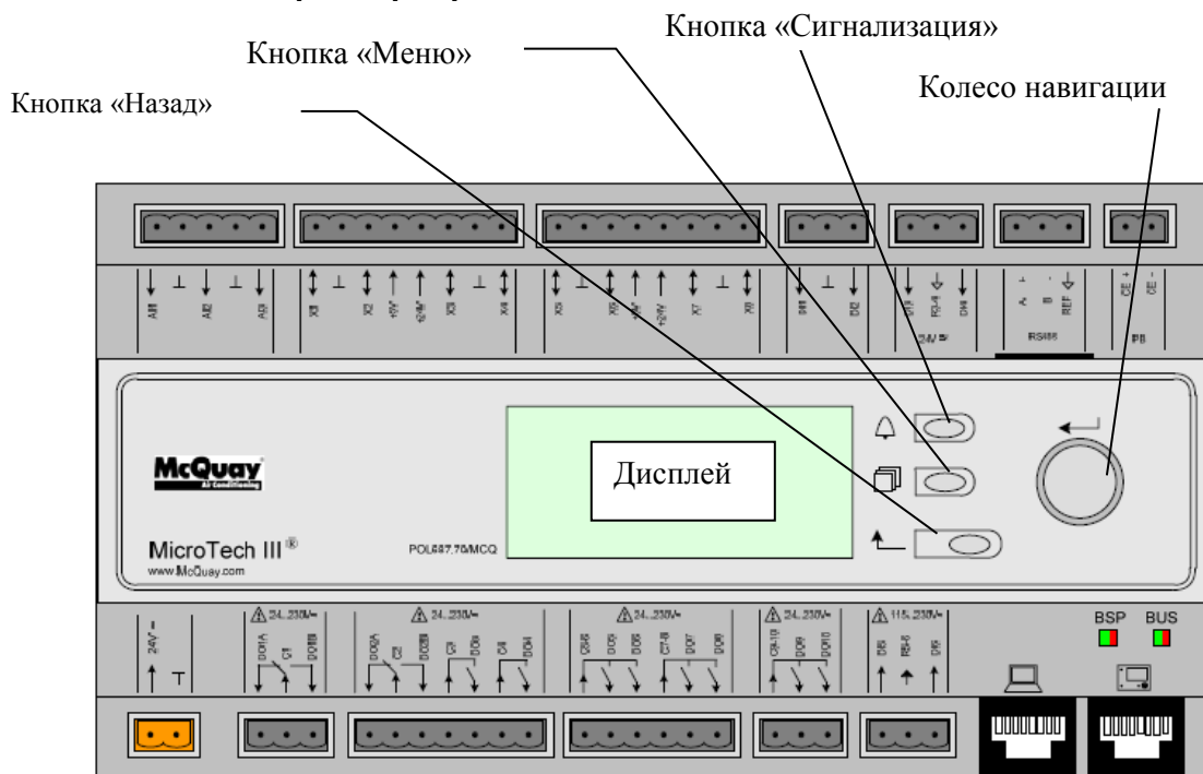
Рис. 6. Контроллер агрегата
