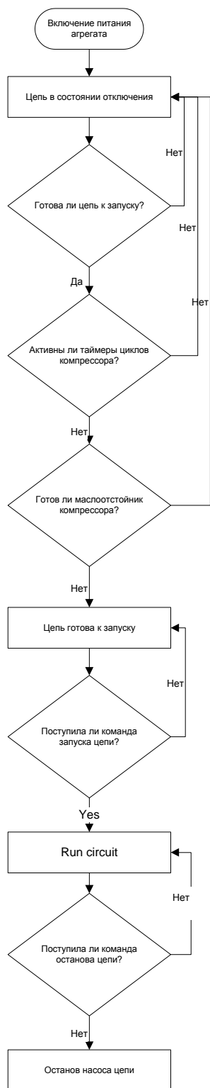
Рис. 5. Порядок работы цепей
