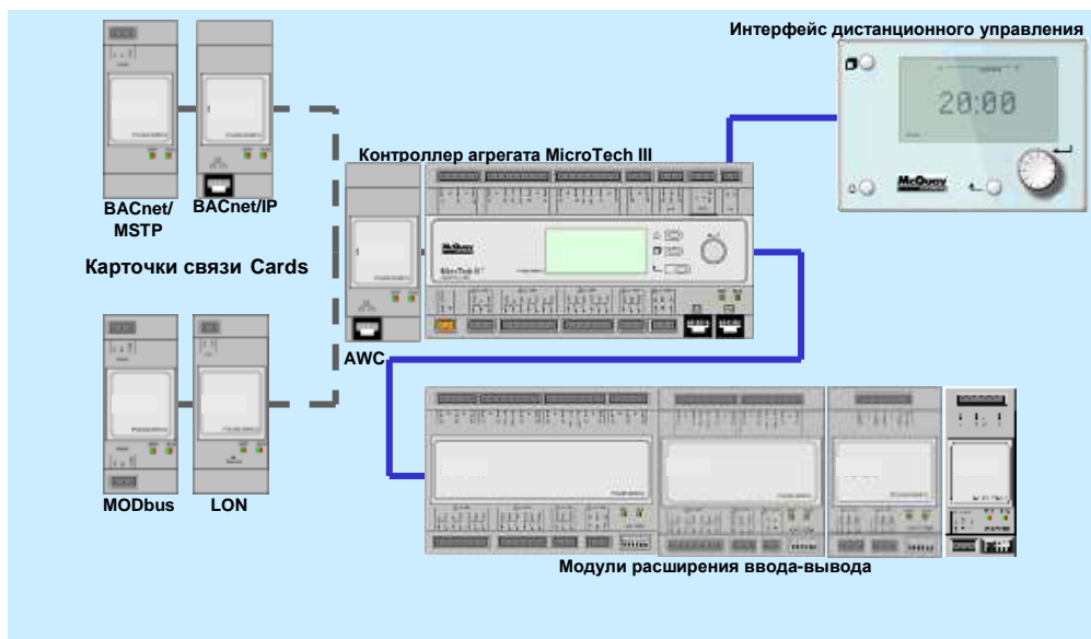
Рис. 3. Аппаратная структура
