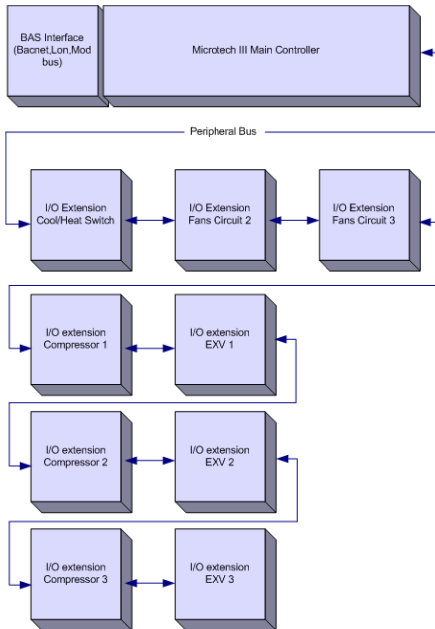
Рис. 3. Архитектура системы
