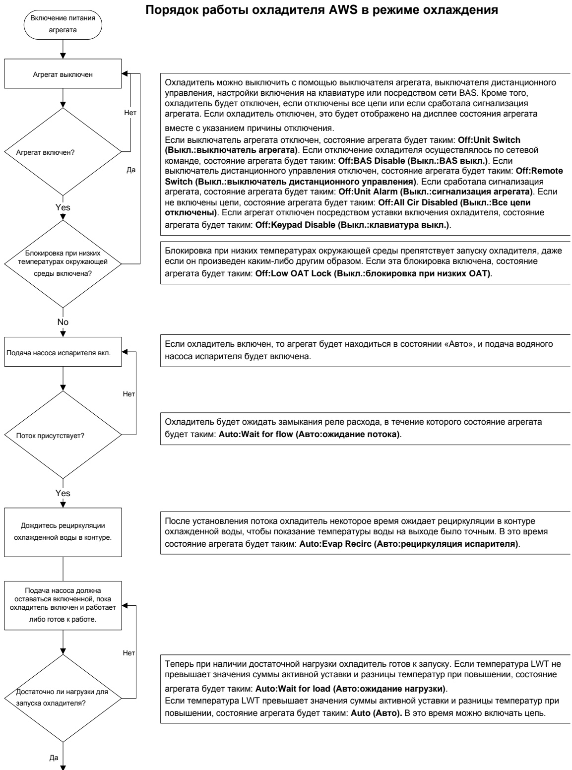
Рис. 5. Порядок работы агрегата (см. рис. 9 для знакомства с порядком работы цепей)
