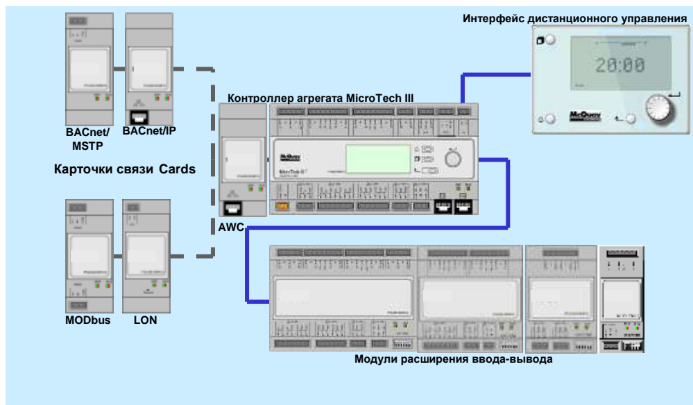
Рис. 6. Аппаратная структура
