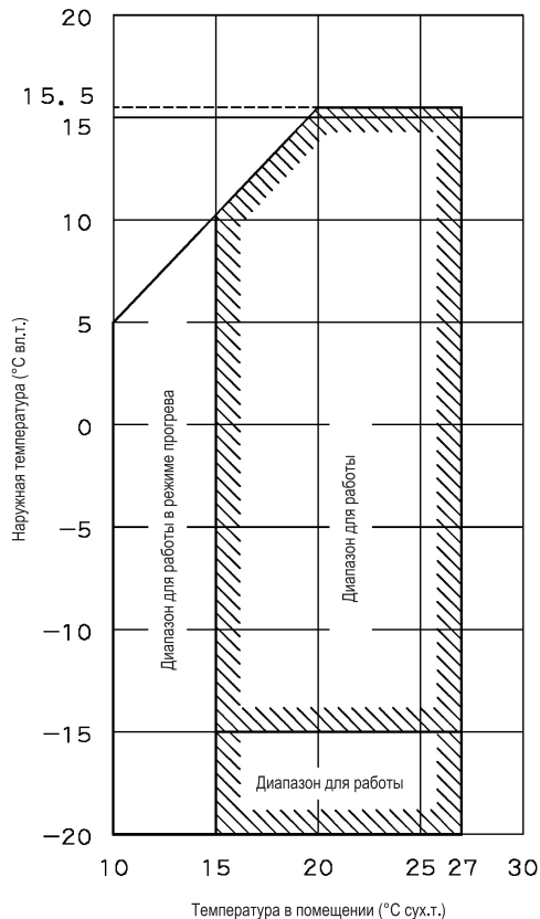
Нагрев
