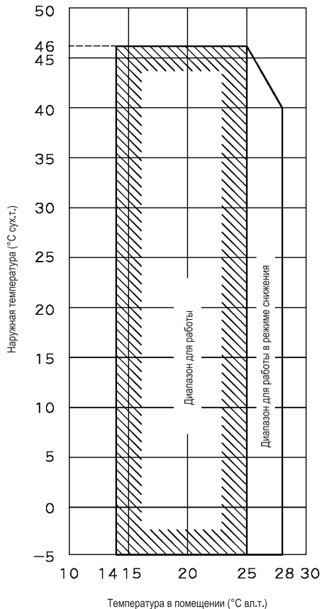
Охлаждение
