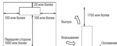
Необходимое место для установки
