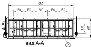
вид А-А
