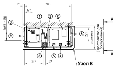
Узел В
