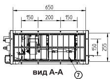
вид А-А
