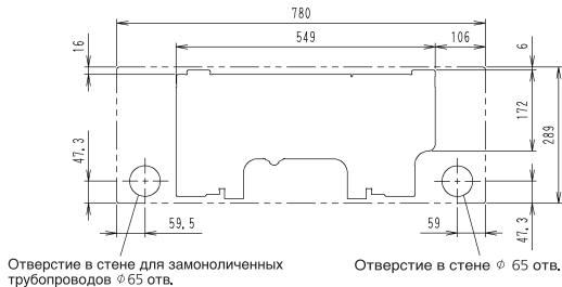
Стандартное расположение отверстий в стене
