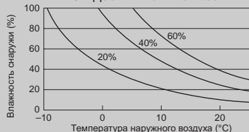
Рис.1 Достижимая влажность
