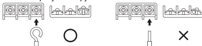
Зачистка проводов на клеммной коробке
