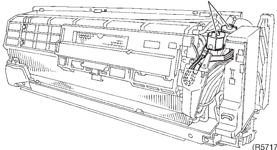
Катушка электромагнитного клапана удаления влаги
